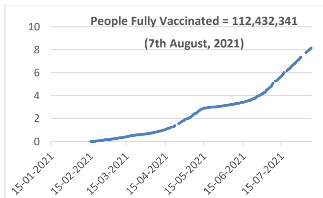
Fig.VI: Fully vaccination per 100 person.
